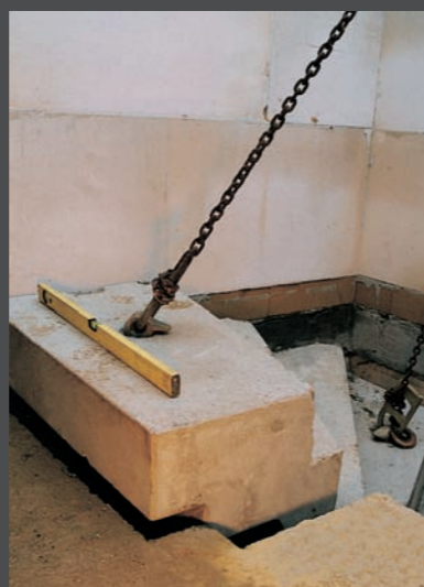
Die Treppen werden im Werk präzise betoniert und in kürzester Zeit auf der Baustelle eingebaut.
